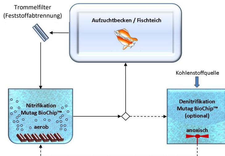
Bild 2: Schema Mutag BioChip 30™ RAS Process
